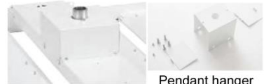
Pendant hanger
